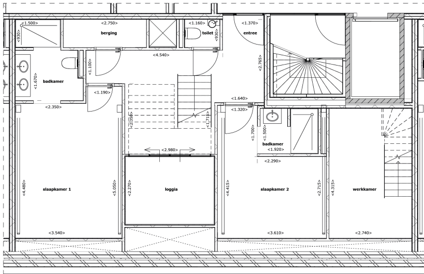
Plattegrond verdieping 03 1:50
