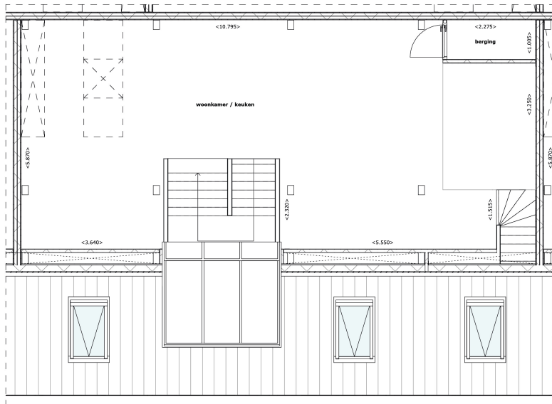
Plattegrond verdieping 04 1:50
